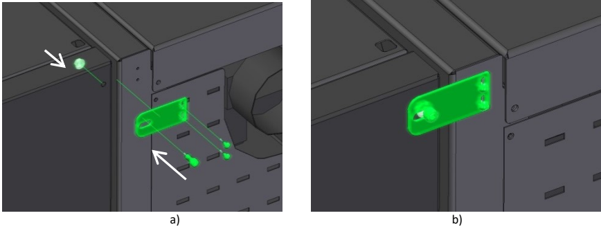
Figura 29 – Fixação traseira do silo à caldeira
