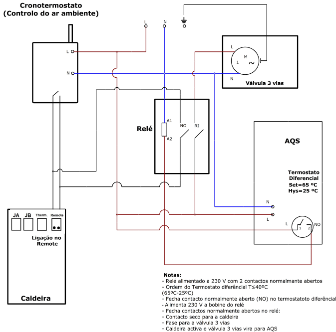
Figura 56 – ligação elétrica de um cronotermostato (controlo do ar ambiente) de um termostato diferencial ligado ao depósito de AQS e da válvula de três vias a uma caixa de relés
