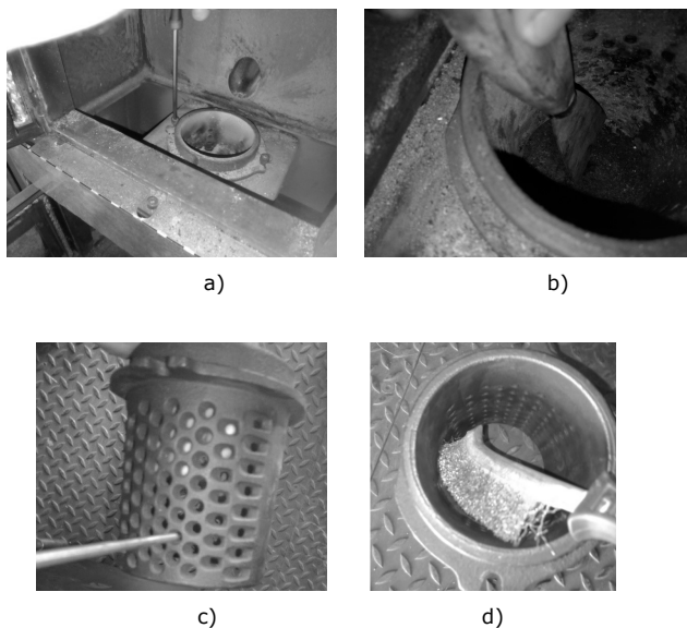
Figura 51 - Limpeza do queimador e do prato de limpeza.
