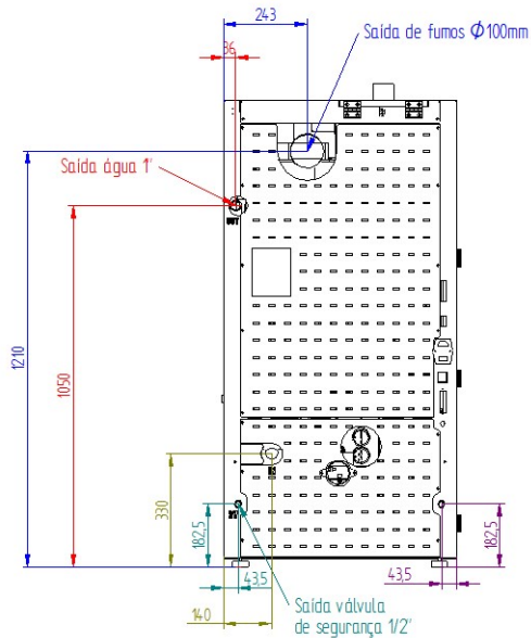
Figura 2 – Ligações hidráulicas da caldeira automáticas a pellets
