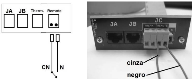
Figura 19 – Ligações do comando externo com fios
