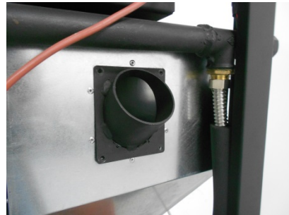
Figura 24 – Montagem da rampa para queda de pellets
