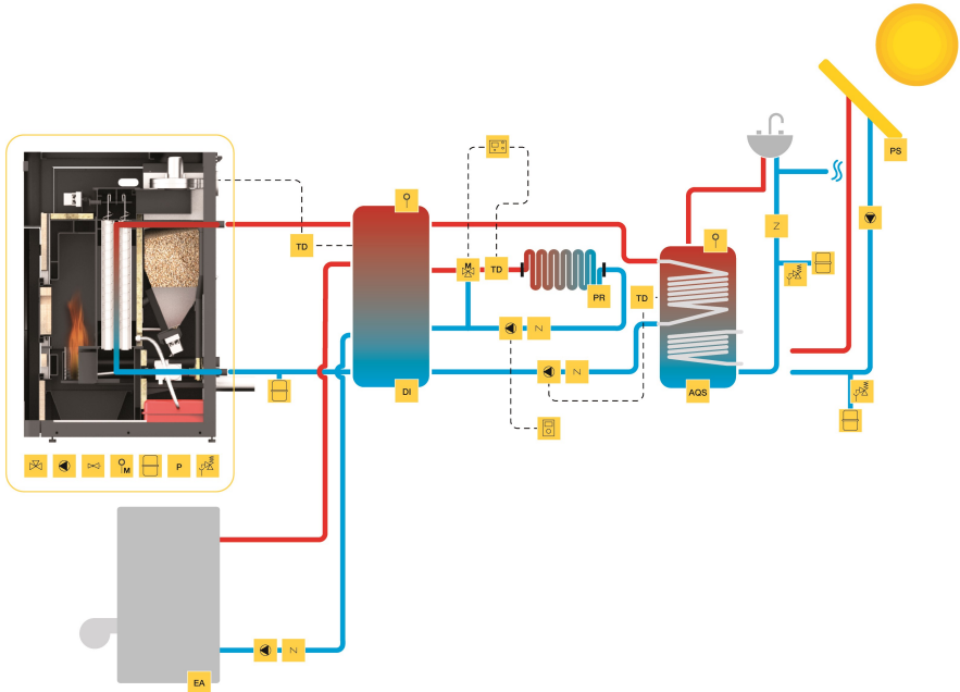
Figure 58 – Ligação a chão radiante, conjugado com outra caldeira de apoio e águas sanitárias combinado com painel solar
