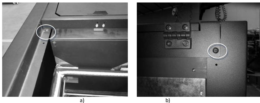
Figura 52 – Retirar os parafusos da tampa superior na parte da frente e na parte traseira da caldeira para ter acesso ao extrator.
