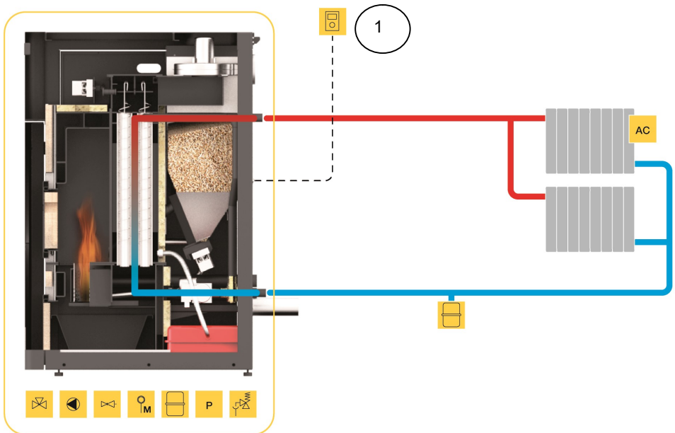
Figura 54 – Ligação simples apenas a radiadores de aquecimento central
