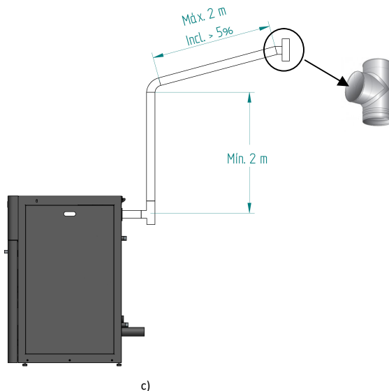
c) Figura 6 – Exemplos de instalações tipo.
