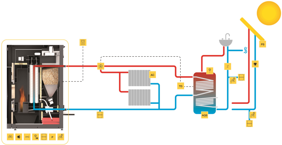
Figura 55 – Ligação a radiadores de aquecimento central e águas sanitárias combinado com painel solar
