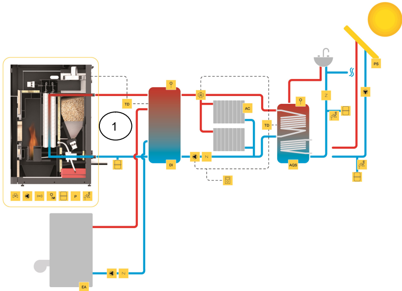
Figura 57 – Ligação a radiadores de aquecimento central, conjugado com outra caldeira de apoio e águas sanitárias combinado com painel solar
