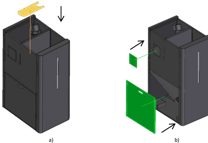
Figura 39 – Colocação do suporte do canal do sem fim e tampas laterais
